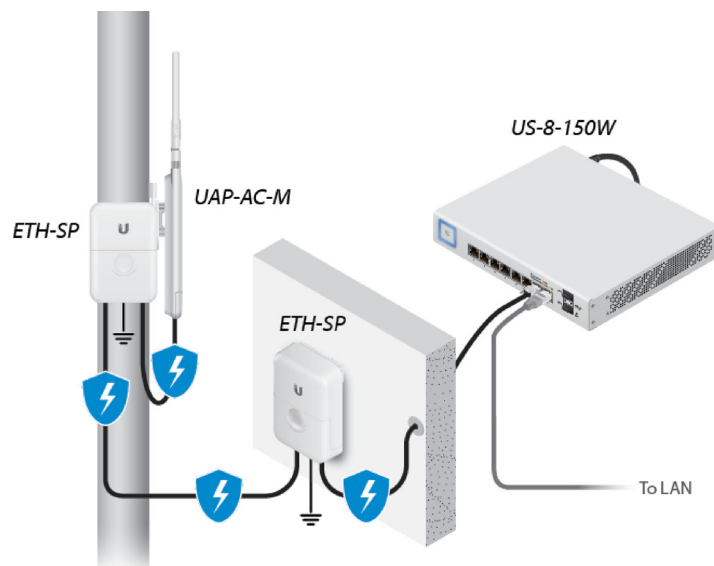
Diagrama que muestra el uso de los protectores contra sobretensiones de Ethernet
